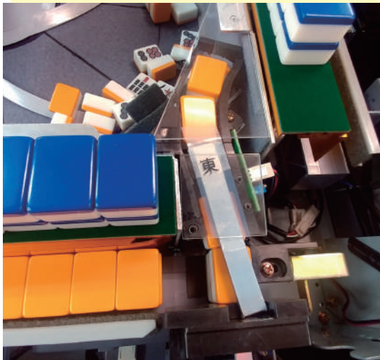
牌整列機構
